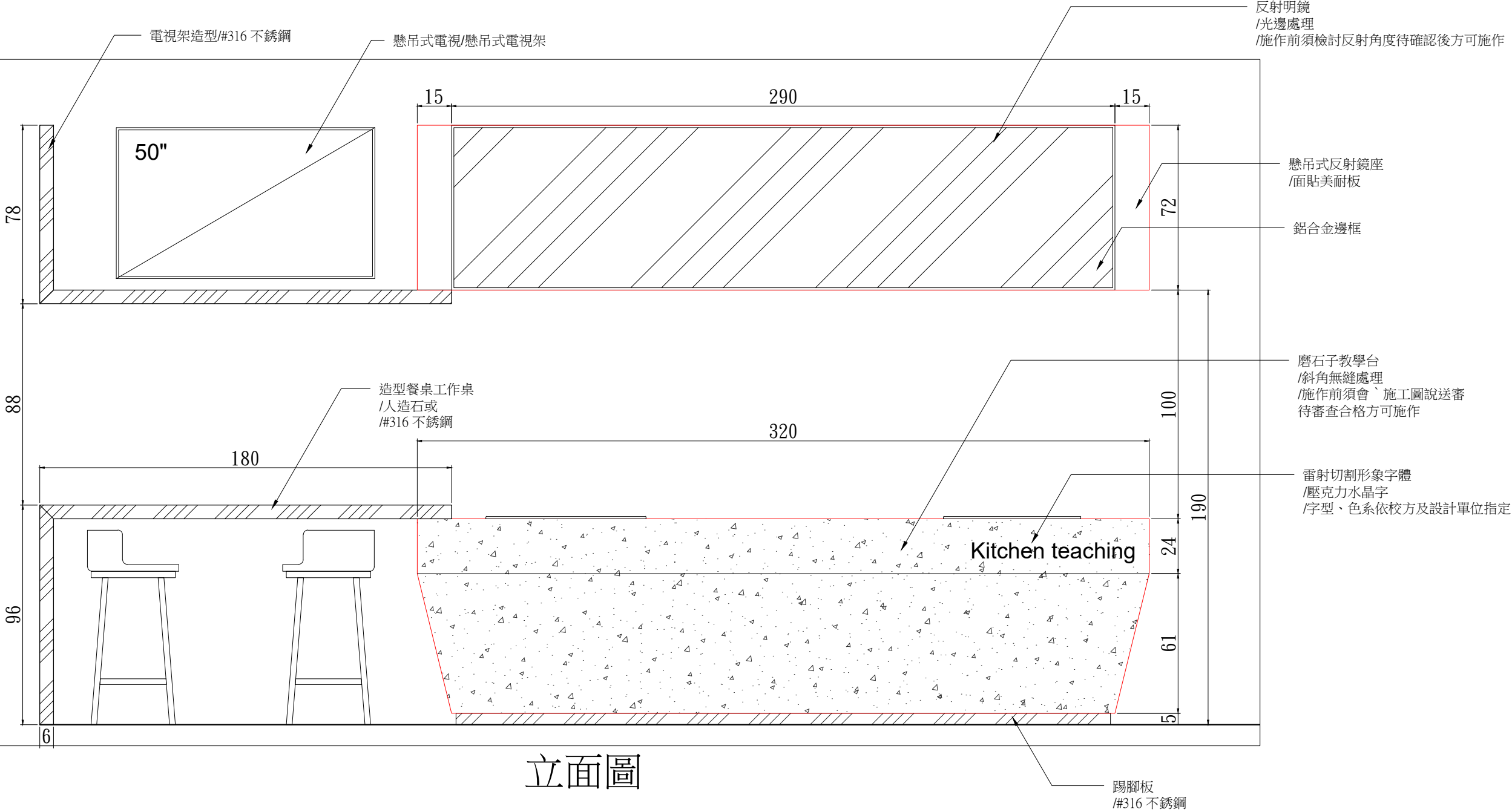
教師檯施工圖 A
